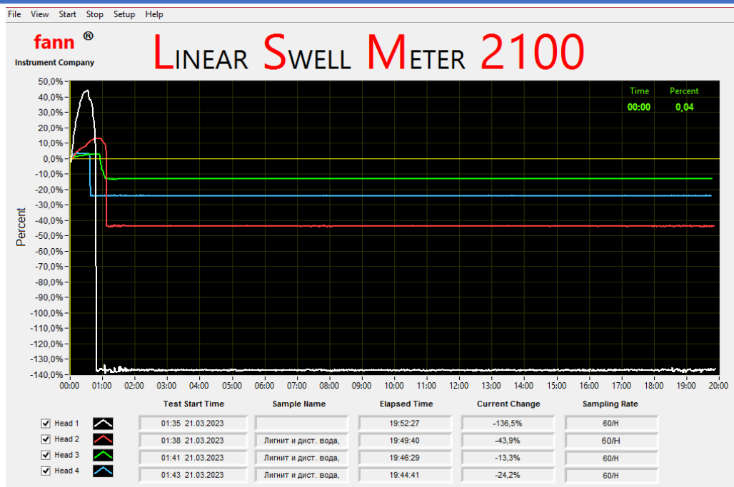
Рис. 8 - Показания прибора LSM 2100 в процессе разрушения искусственно созданных образцов обвальнoй породы в 1% растворе ФХЛС и 1% растворе органофильного лигнита
