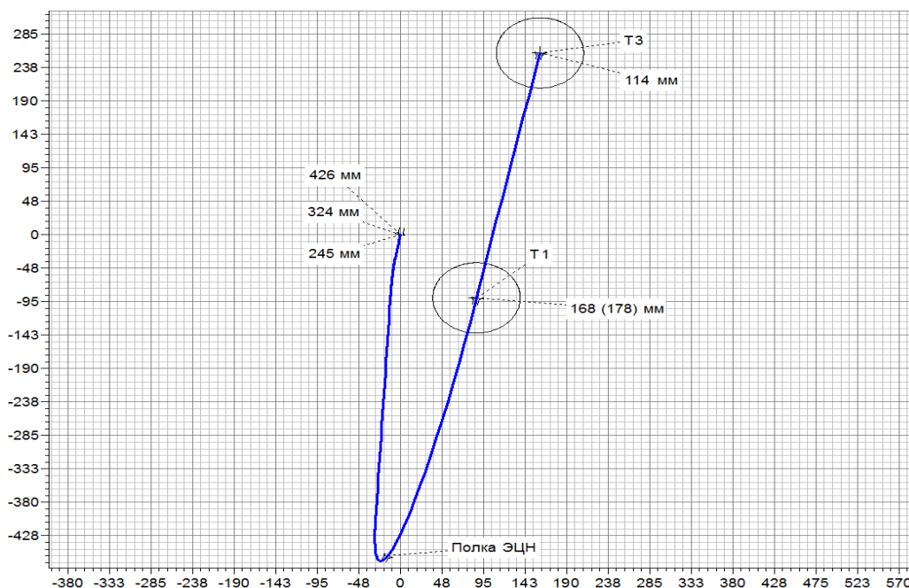
Рисунок 4 – Горизонтальная проекция профиля скважины с отрицательным отходом и разворотом по азимуту
