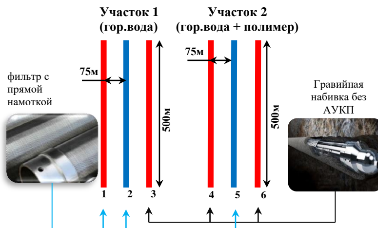
Рис.1 – принципиальная схема ОПР
