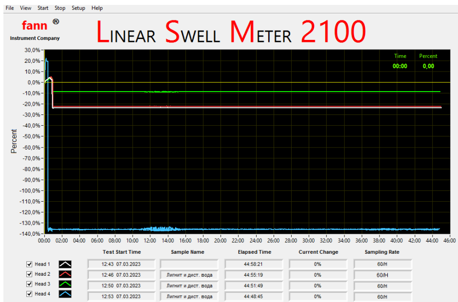
Рис. 5 - Показания прибора LSM 2100 в процессе разрушения искусственно созданных образцов обвальная породы в 1% растворе органофильного лигнита
