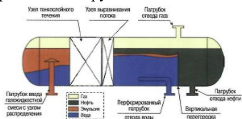
Рис.2 Принципиальная схема модернизированного ТФС
