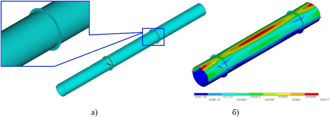
Рис.1. Геометрическая модель и фрагмент конечно-элементной сетки а) и расчетное смещение узлов б) сборного стеклопластикового футляра.
