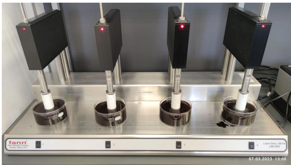
Рис. 3 - Фото прибора LSM 2100 в процессе испытания искусственно созданных образцов обвальнй породы в 1% растворе органофильного лигнита
