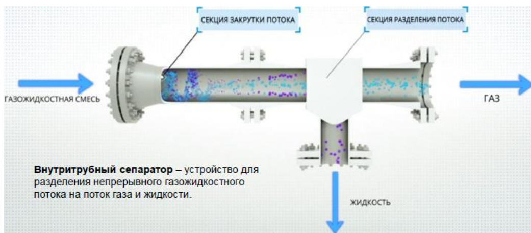
Рисунок 2. Принцип работы внутритрубного сепаратора.
