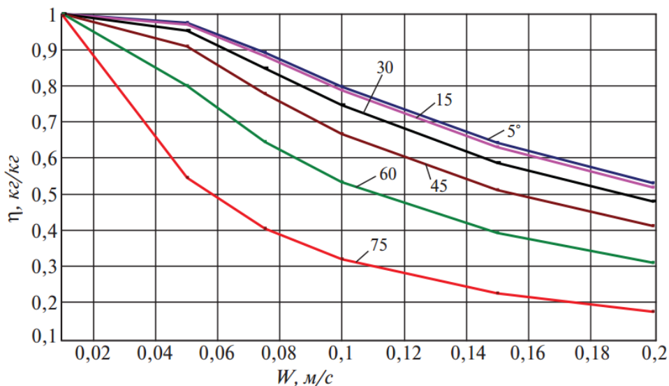
Рис. 2. Зависимость эффективности \eta сепарации капель от скорости W потока сплошной фазы при разных углах наклона гофрированных пластин в пакете интенсифицирующей насадки
