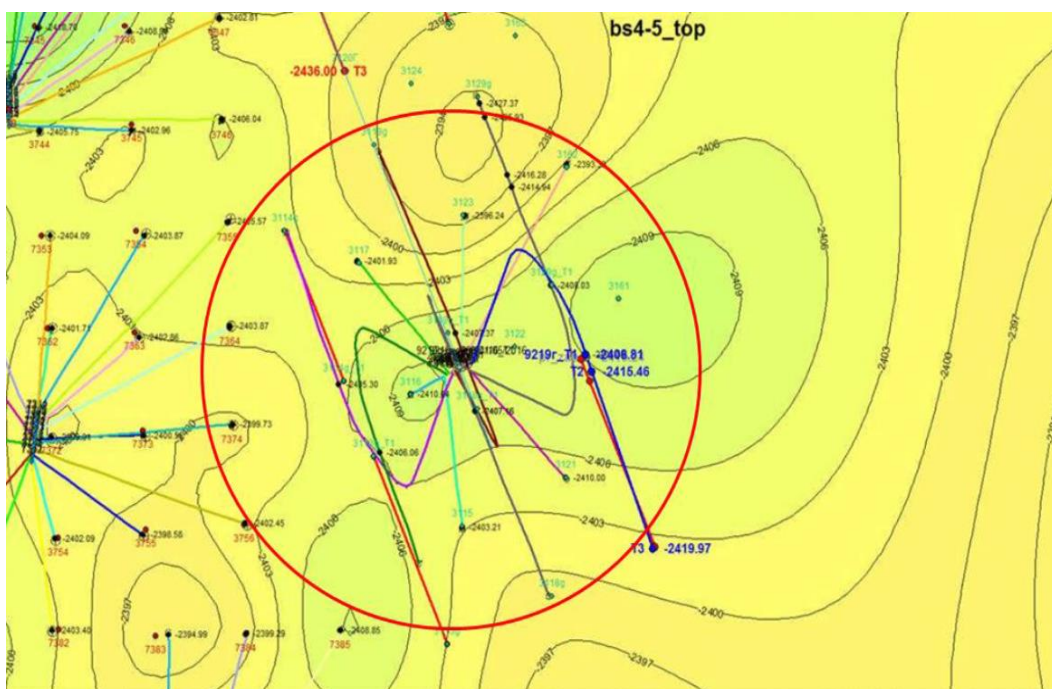
Рисунок 1 – Кустовая площадка с условной окружностью по точкам Т1, Т2, Т3
