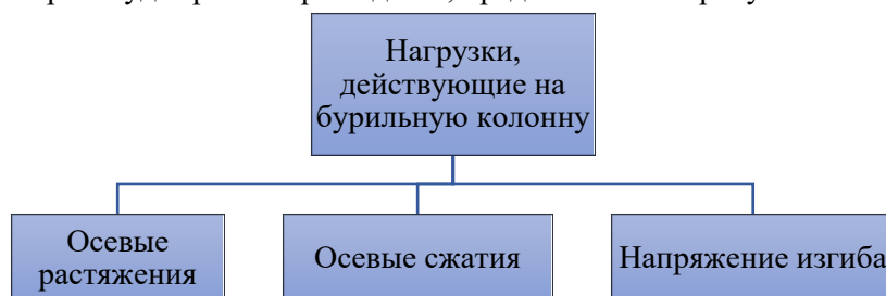
Рисунок 1 - Нагрузки, действующие на бурильную колонну
