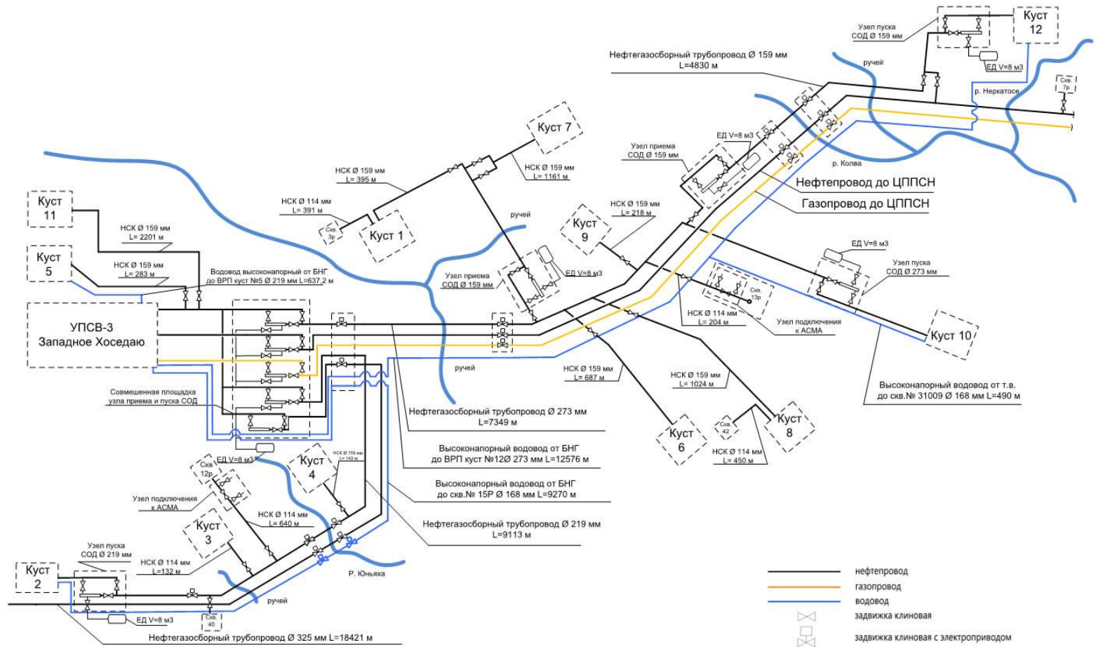
Рис.1 Принципиальная схема системы сбора и транспорта продукции со скважин Западно-Хоседаевского месторождения
