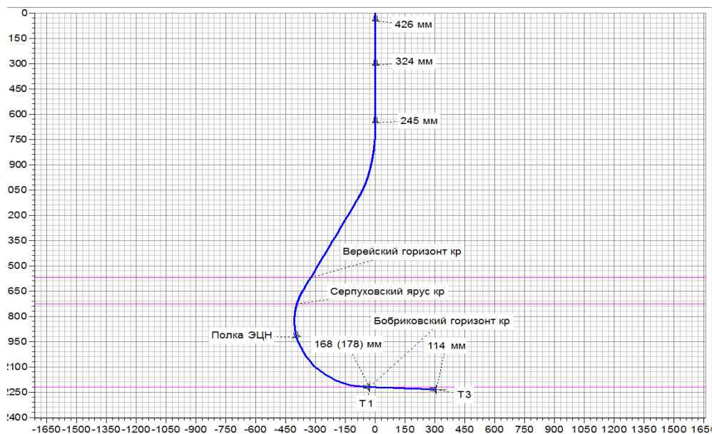
Рисунок 3 – Вертикальная проекция профиля скважины с отрицательным отходом
