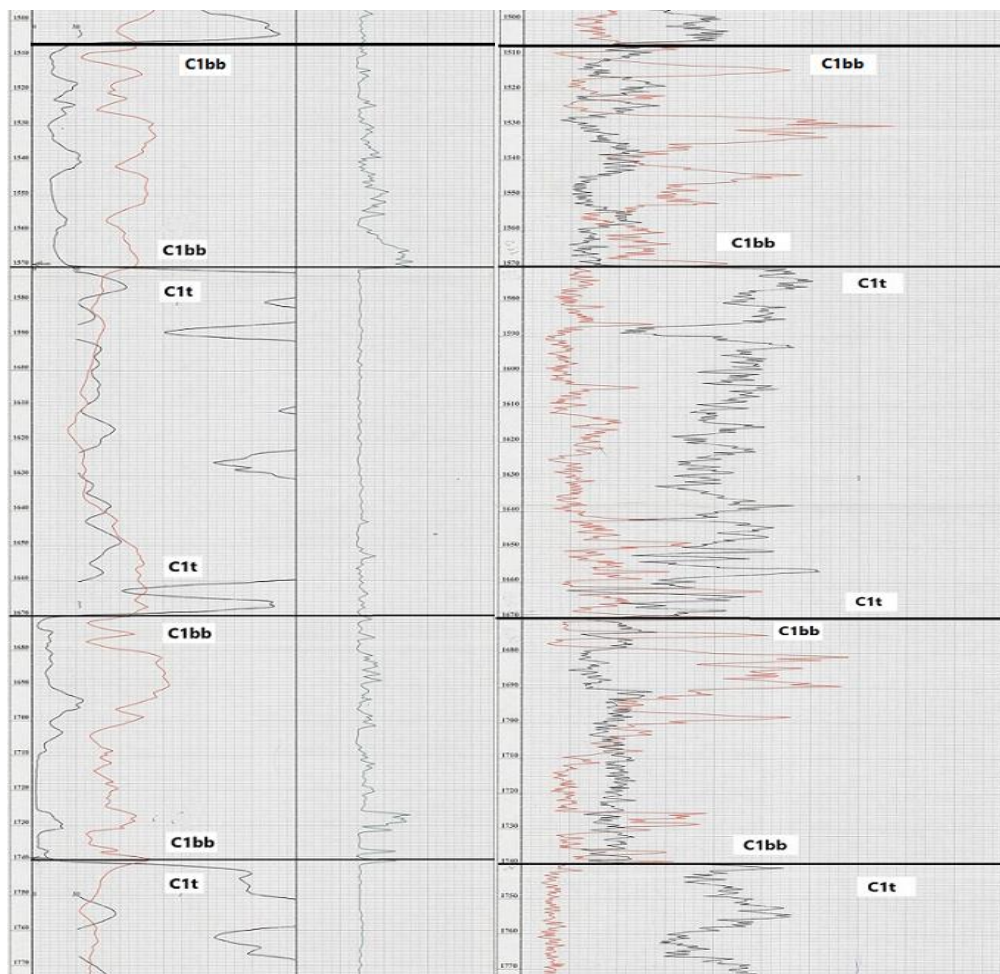
Рисунок 3 – Стандартный каротаж, калвернометрия, радиоактивный каротаж в зоне тектонического разлома скважины №10
