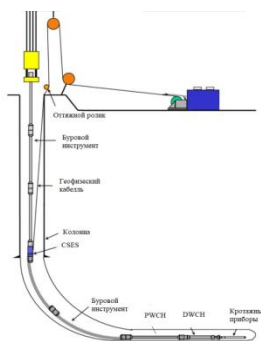
Рис.7 Проведение каротажа на бурильных трубах.
