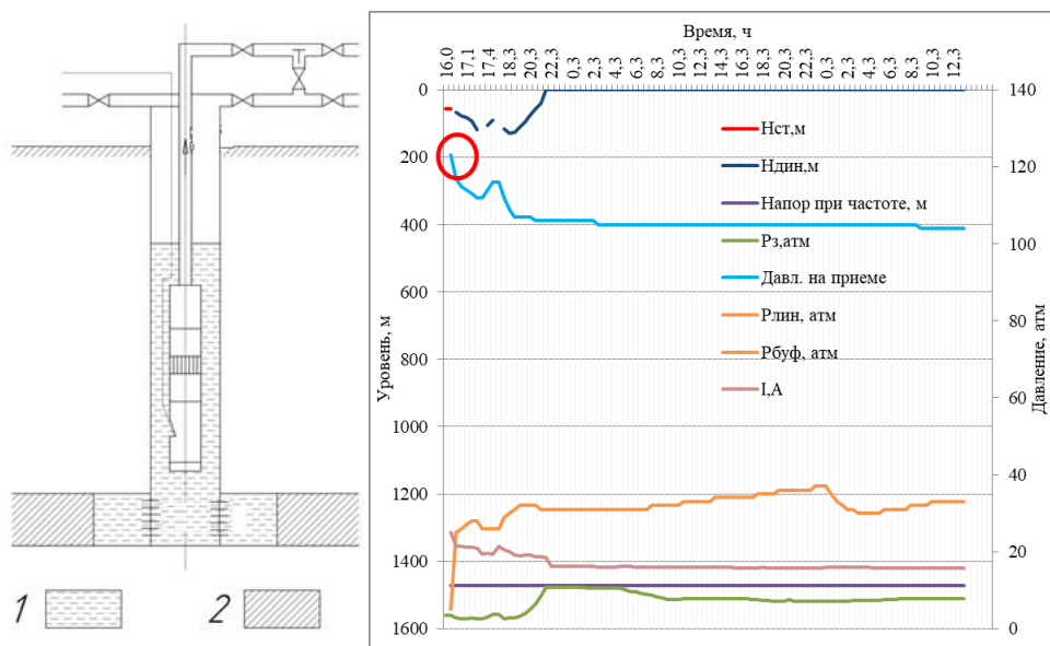
Рисунок 1 - Конструктивная схема скважины с УЭЦН и карта ВНР 1 - жидкость глушения, 2 - пластовая жидкость
