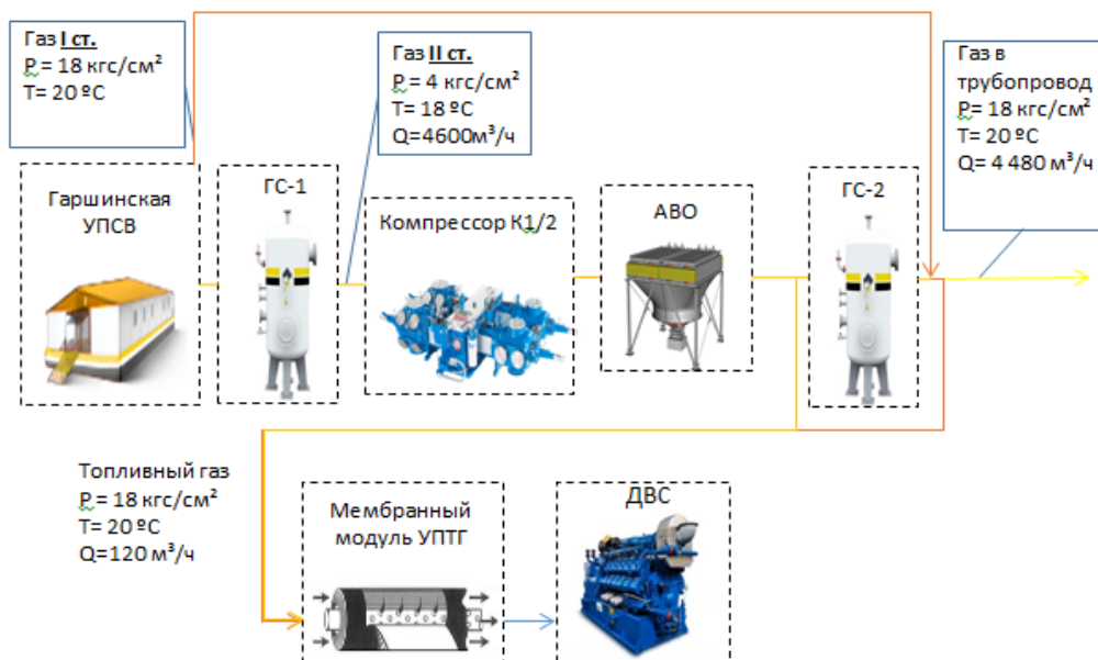
Рис. 1. Принципиальная схема Гаршинской ГКС
