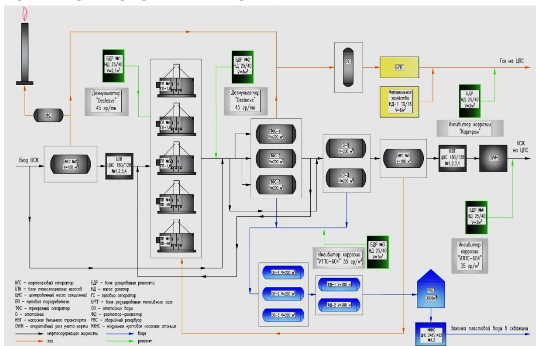
Рис.1. Принципиальная схема УПСВ – 3
