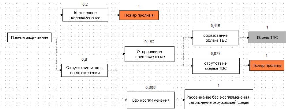
Рис. 3 - Логическая схема развития аварии, связанной с выбросом горючего вещества из газового сепаратора, отстойника
