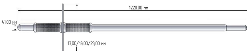
Рис.5 Расходомер с тепловым импульсом HFP-2293
