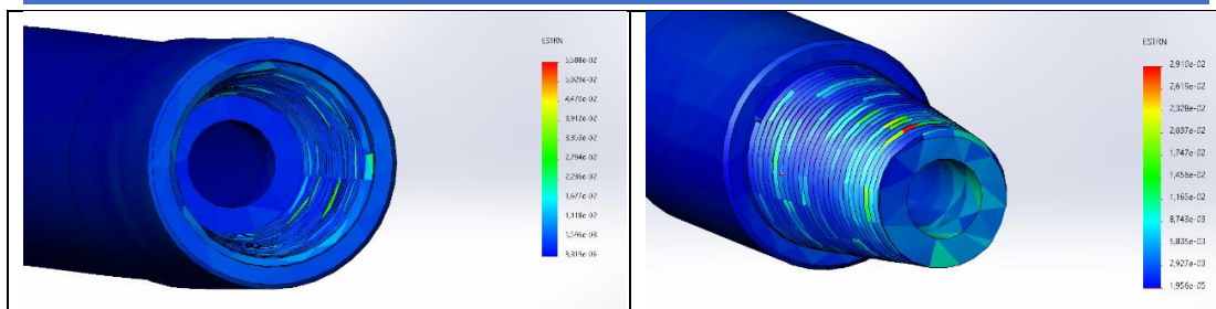
Рисунок 9 - Величины деформации ниппеля и муфты, возникающих при изгибающих нагрузках
