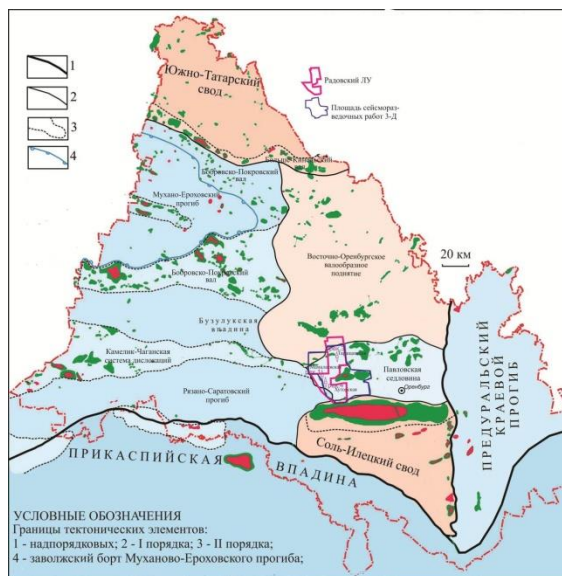
Рисунок 1 - Фрагмент из обзорно-тектонической схемы Оренбургской области [1].
