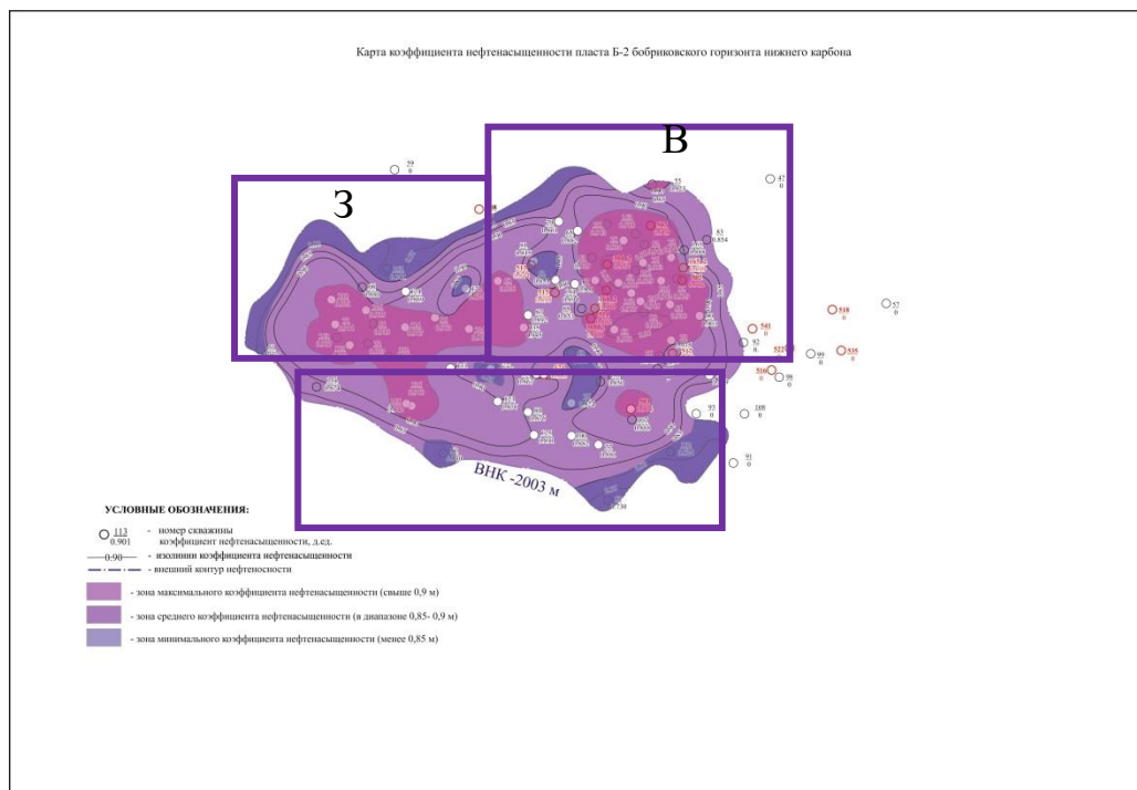
Рис 3. Карта коэффициента нефтенасыщенности
