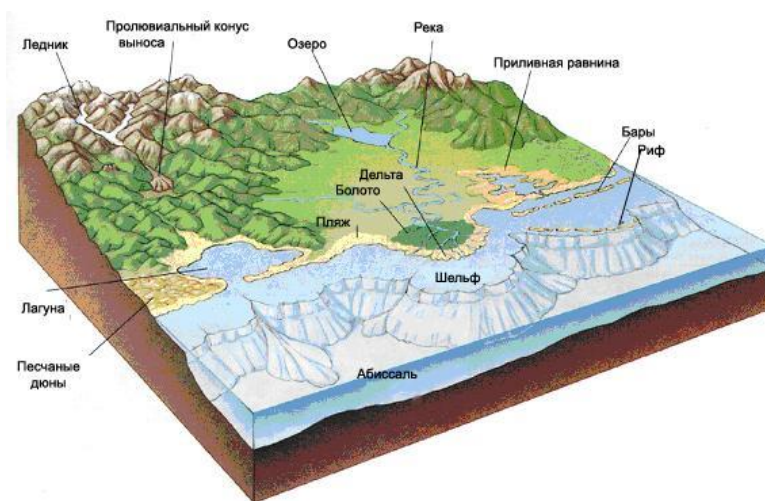
Рисунок 2 - Блок схема континентальной зоны осадконакопления [4]
