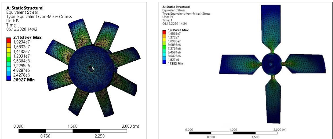
Рисунок 1 – Сравнение напряжений в рабочих колесах АВО (слева из стали, справа из композитов)
