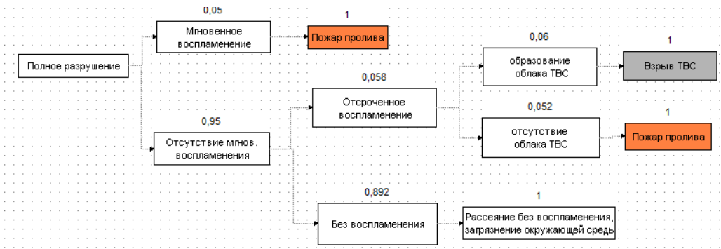
Рис. 2 - Логическая схема развития аварии, связанной с выбросом горючего вещества из РВС
