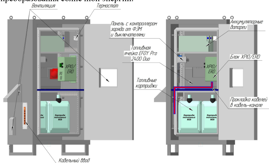
Рисунок 3. Автономный комплекс электроснабжения (АКЭ) с блоком сбора данных.
