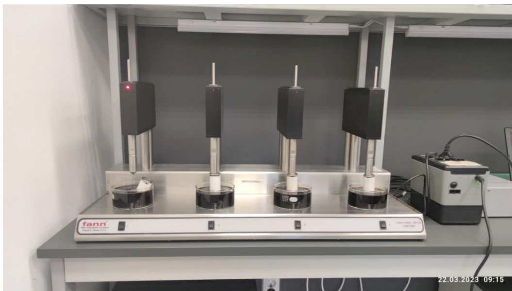
Рис. 7 - Фото прибора LSM 2100 в процессе разрушения искусственно созданных образцов обвальнй породы в 1% растворе ФХРС и 1% растворе органофильного лигнита
