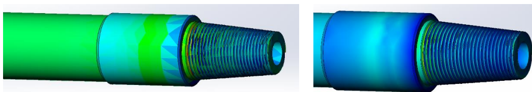
Рисунок 6 - Величины деформации и напряжения, возникающих при растяжении ниппеля замкового соединения
