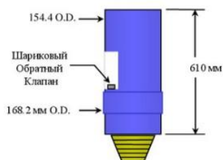
Рис.6 Разрезной переводник CSEC
