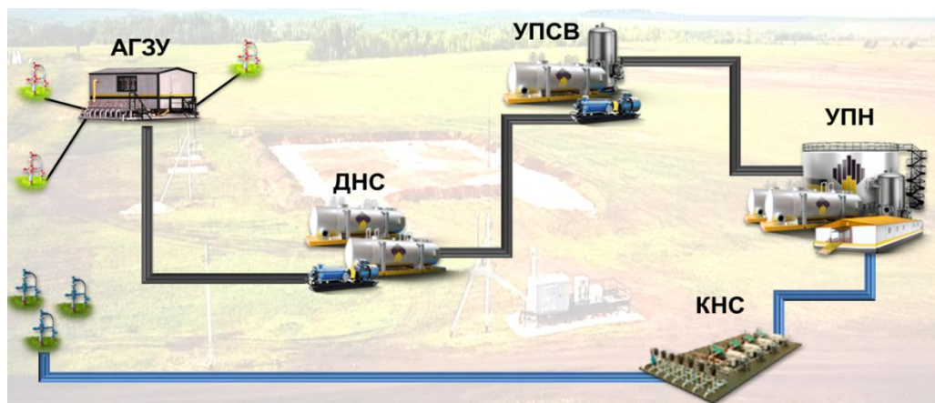
Рис.2 Система сбора и транспорта нефти
