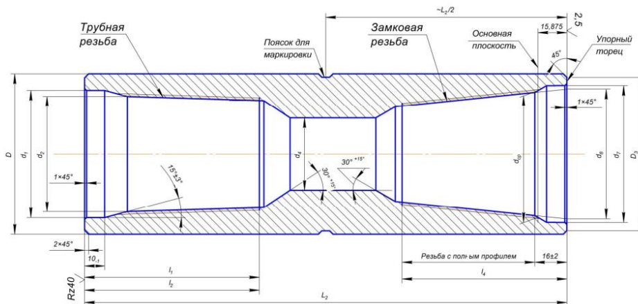
Рисунок 3 - Чертёж муфты замков типов ЗН, ЗШ и ЗУ
