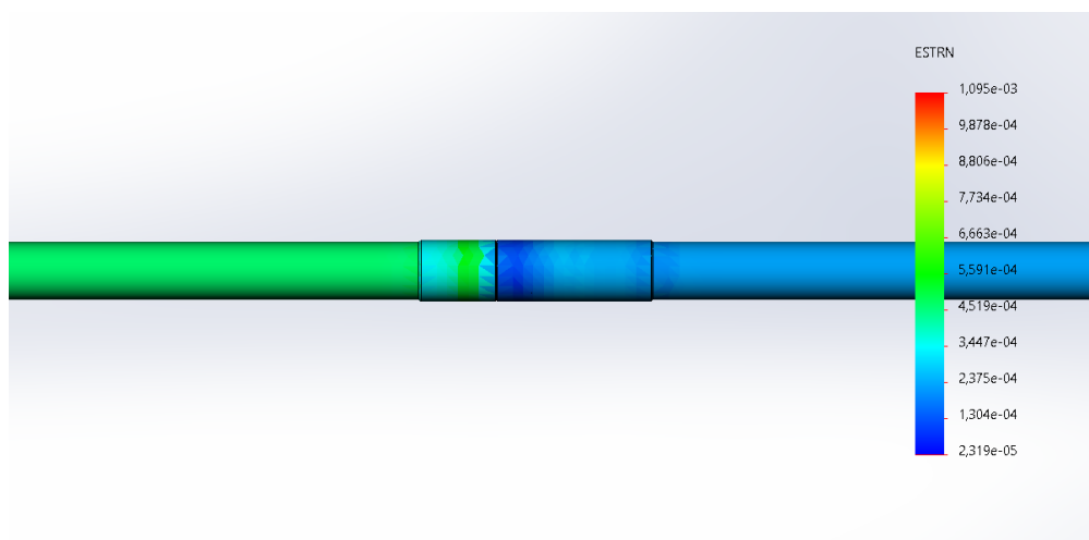
Рисунок 5 - Величины деформаций, возникающих при растяжении замкового соединения
