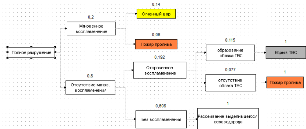
Рис. 3 - Логическая схема развития аварии, связанной с выбросом горючего вещества из газового сепаратора, отстойника
