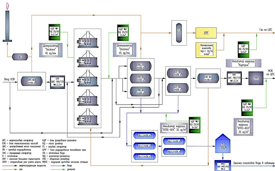
Рис.1. Принципиальная схема УПСВ-3
