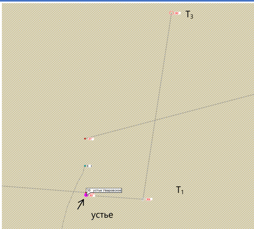
Рисунок 2 – Одиночная горизонтальная скважина с отрицательным отходом по точкам T1 и T3
