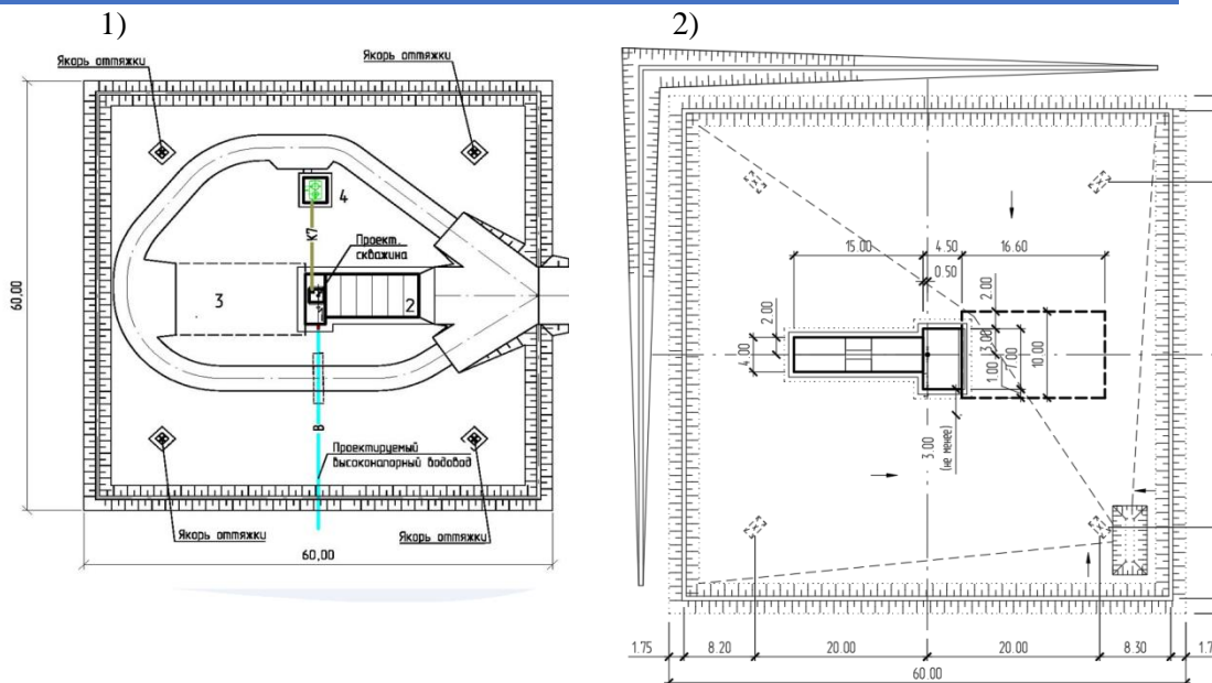
Рис. 2 Типовая схема расстановки площадок и оборудования (1) и оптимизированная схема (2) при обустройстве нагнетательной скважины Оренбургской области
