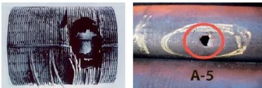
Рисунок 1 - Эрозия внутрискваженного оборудования
