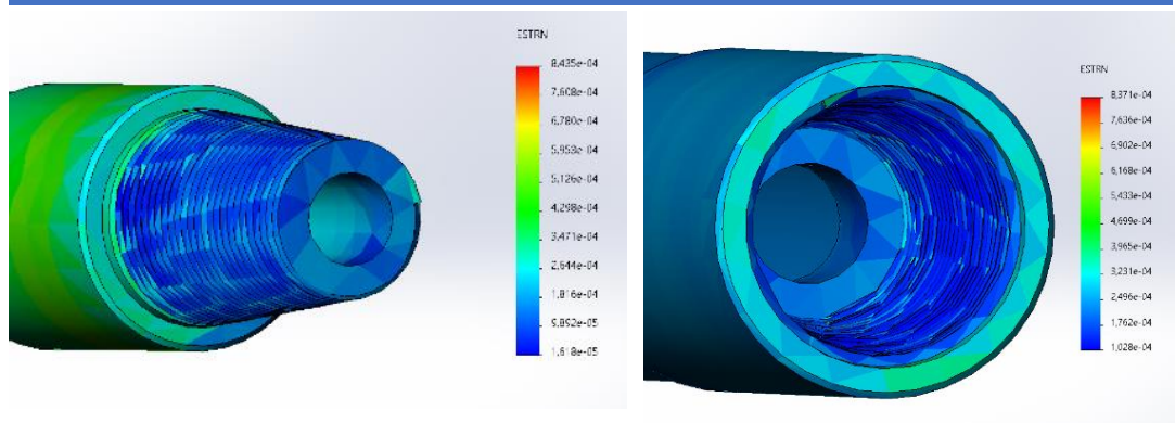
Рисунок 8 - Величины деформации муфты и ниппеля, возникающих при сжатии замкового соединения
