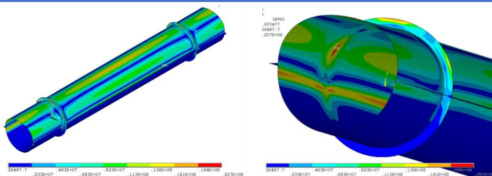
Рис.2. Напряжения в сборном стеклопластиковом футляре
