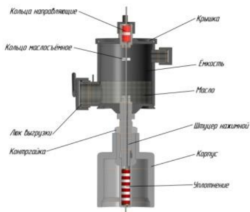
Рис. 2 – Сальниковое устройство лубрикатора[9].
