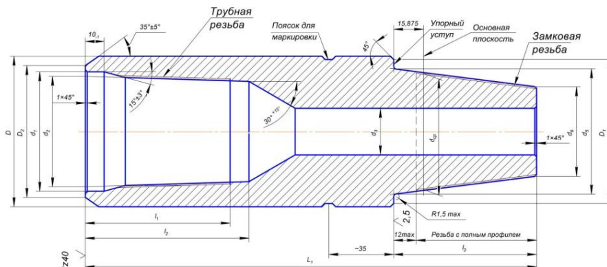
Рисунок 2 - Чертёж ниппеля замков типов ЗН, ЗШ и ЗУ
