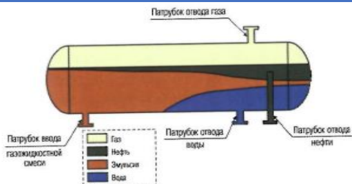
Рис.1 Принципиальная схема работы ТФС
