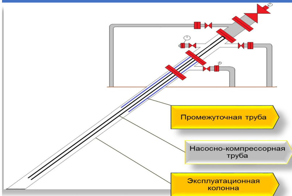
Рис.3 Шурф предварительного сброса воды (ШПСВ)
