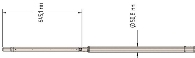
Рис.4 Пробоотборник глубинный BHFS
