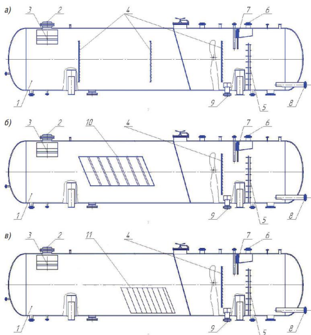
Рис.3. Принципиальные конструкции реконструированных трехфазных сепараторов
