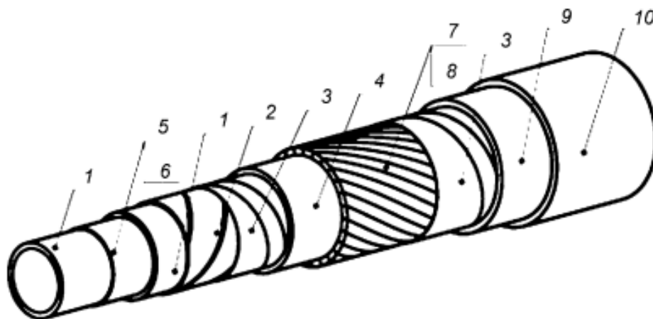
Рисунок 2 - пример конструкции ПАТ с армирующим слоем из нитей, проволоки, корда
