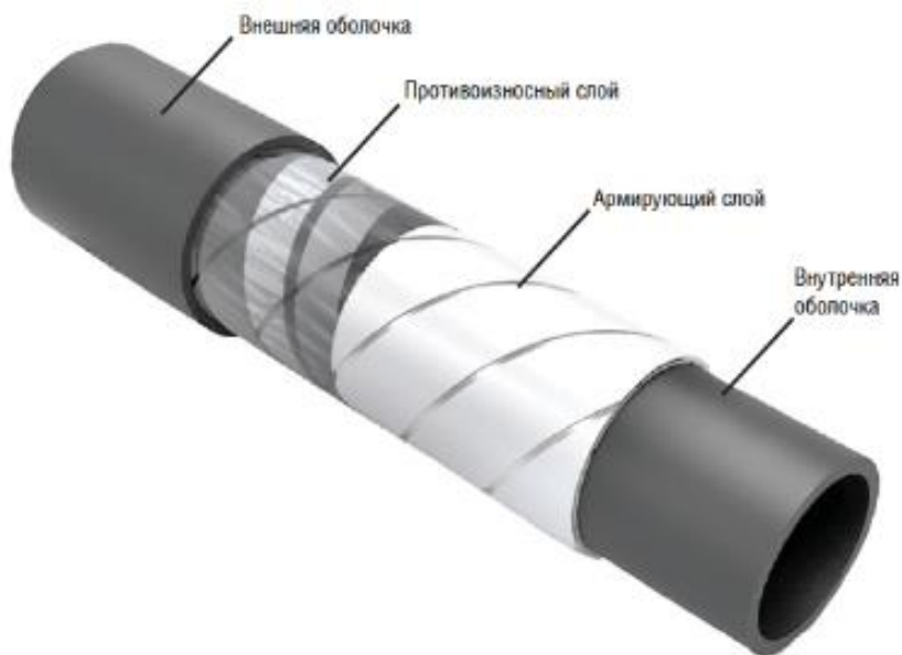
Рисунок 1 – Принципиальная схема ПАТ
