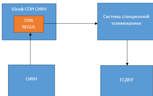
Рисунок 1 – блок-схема СОИ СИКН
