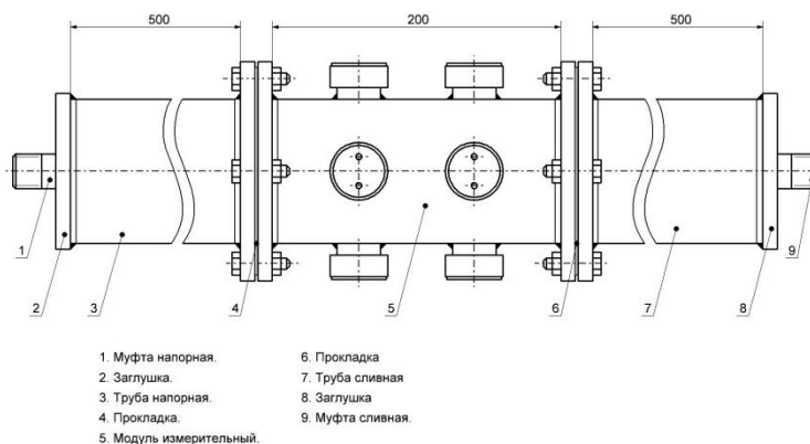
Рис.1 Эскиз выкидной линии трубопровода
