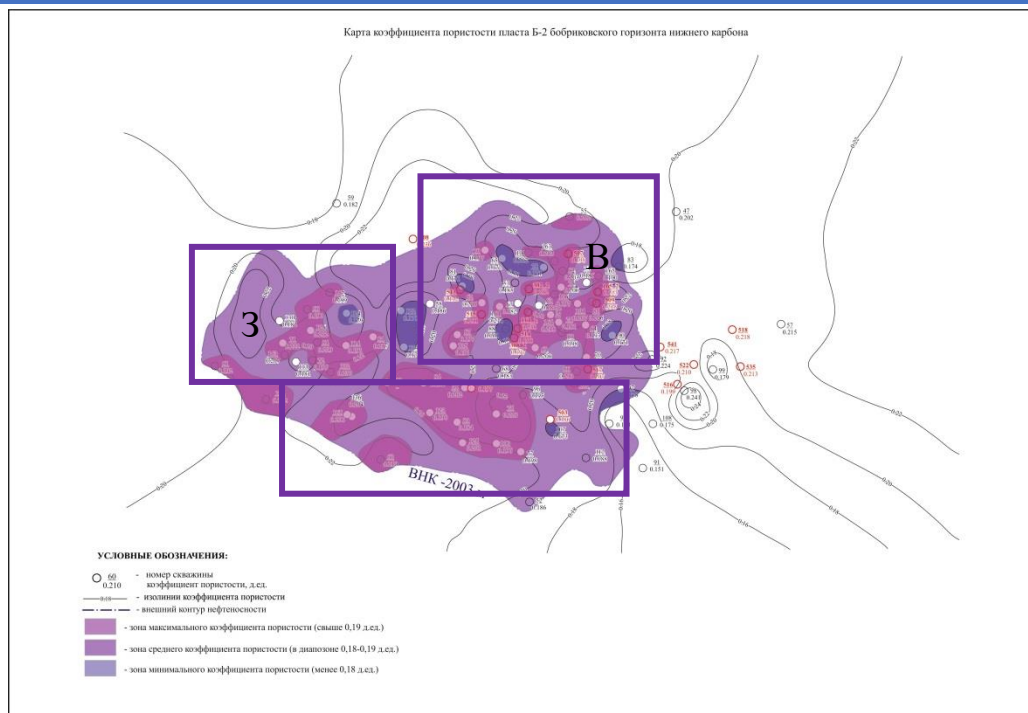
Рис 2. Карта коэффициента пористости
