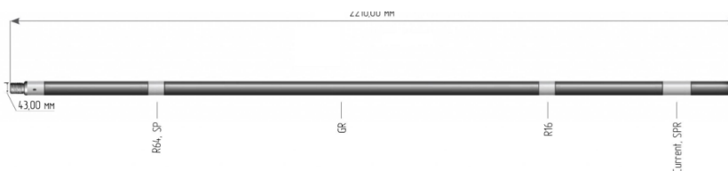
Рис. 1 Прибор электрического и гамма каротажа 40GRP-1000
