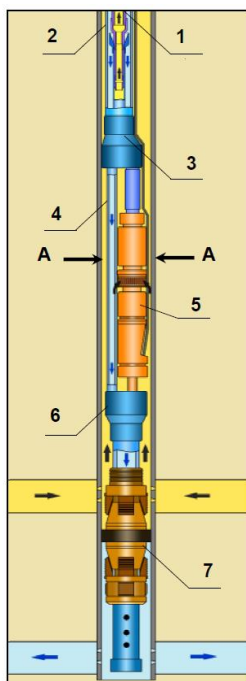
Рисунок 1 – Схема подземного оборудования скважины
